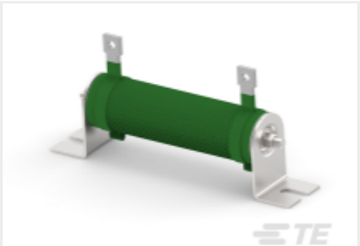
TE 产品编号 CAT-C339-T2201 线绕电阻器：矿物，2.5 Kw
