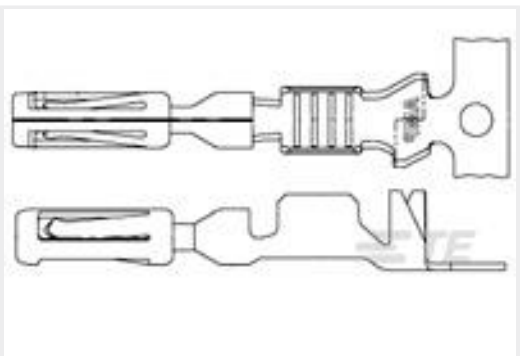
TE 产品编号 770520-1 AMPSEAL, TERMINAL, TIN PLATE, 16-20AWG WIRE
