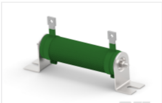
TE 产品编号CAT-C339-T2201 线绕电阻器：矿物，2.5 Kw
