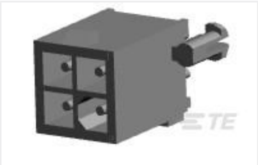
TE 产品编号1-770174-1 04P MINI UMNL ASSY VO SNAU LF
