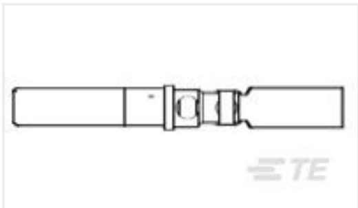
TE 产品编号692485-000 D-602-0289
