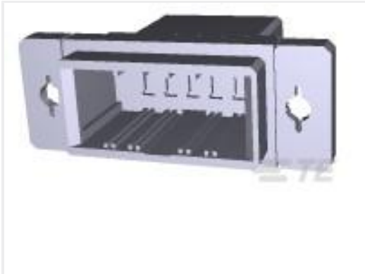
TE 产品编号178803-5 DYNAMIC D3100D TAB HSG PM 10P
