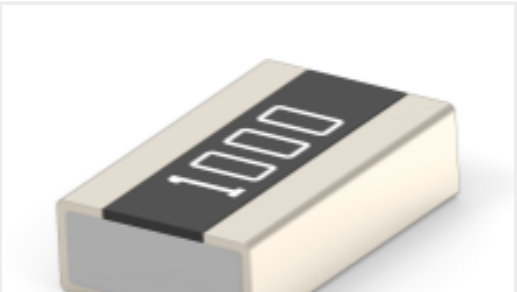
TE 产品编号1-2176554-2 3430 A2 1% 2R7 150ppm 1k RL
