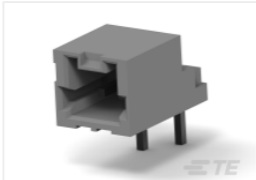
TE 产品编号 292206-2 MINI CT SGL DIP H 2P NAT
