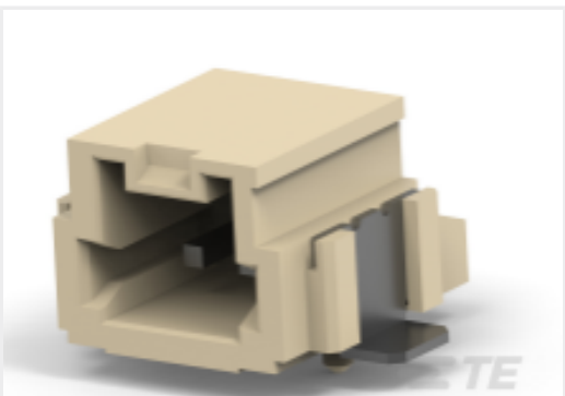
TE 产品编号 292227-2 1.5 MINI CT SGL H SMT W BOSS 2
