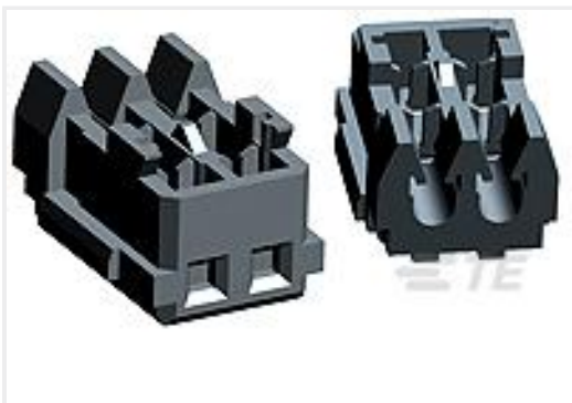
TE 产品编号 292271-2 MT REC ASSY AU-PL. 2P GRAY
