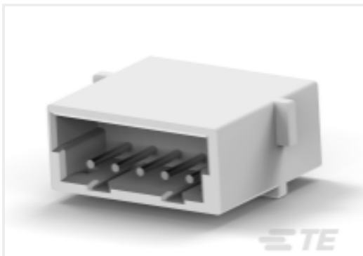
TE 产品编号 CAT-3980655-RHAFH CT 继电器公端组件：自由悬挂
