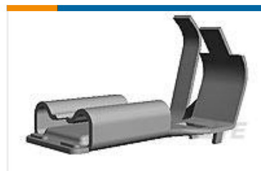
TE 产品编号175019-1 187 PL EX FLAG REC. 22-16AWG PTBR
