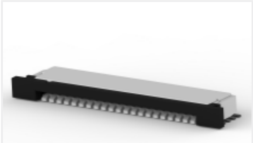
TE 产品编号 2-84952-0 1MM FPC HORZ.BTTM CONT.ASS.20P
