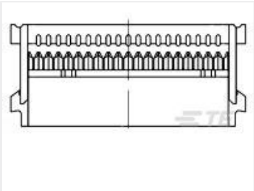
TE 产品编号2-1658526-9 609-1630LF=FSKT IDC S 16 30AU
