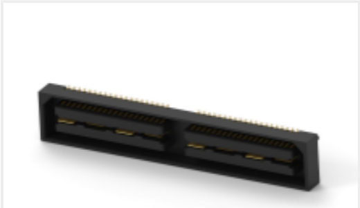
TE 产品编号 6-1658012-2 MSB0.80RC-ASY080FL,GP,10,-TR
