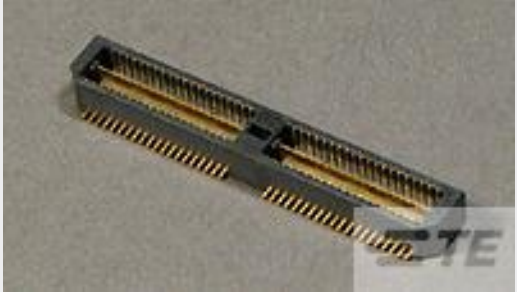
TE 产品编号 1658044-2 MSB0.80PL5ASY080FL,-,F,-TY
