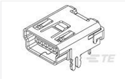
TE 产品编号2172034-1 MINI USB B, RCPT, R/A, T/H, PBT, Tray
