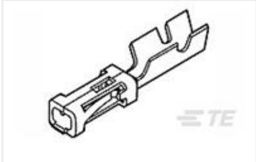
TE 产品编号2-87195-5 MOD IV RECP LP
