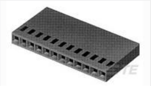
TE 产品编号87499-8 04 MODIV HSG COMP SR .100CL
