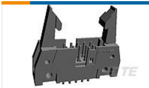
TE 产品编号1-5499923-0 A/L UNIV HDR 50P VERT LG LAT
