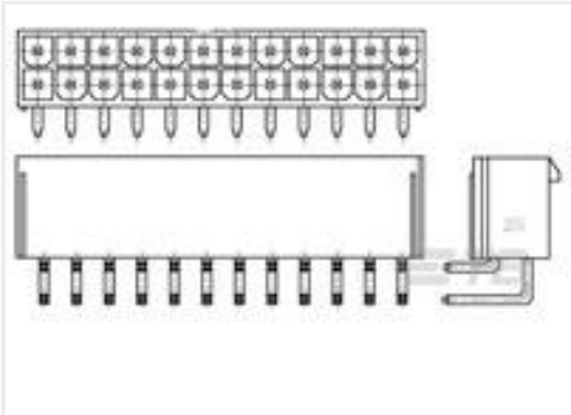
TE 产品编号1586041-2 2P VAL-U-LOK R/A HDR V2
