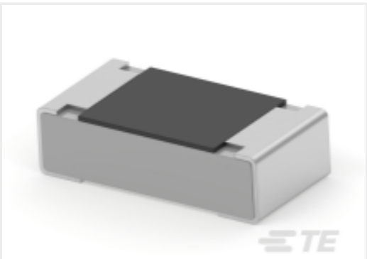
TE 产品编号2-2176340-6 CRGCO 0603 15K 5%
