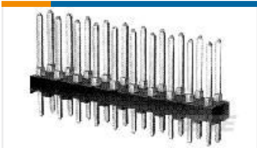
TE 产品编号1-87227-0 20 MODII HDR DRST UNSHRD .100
