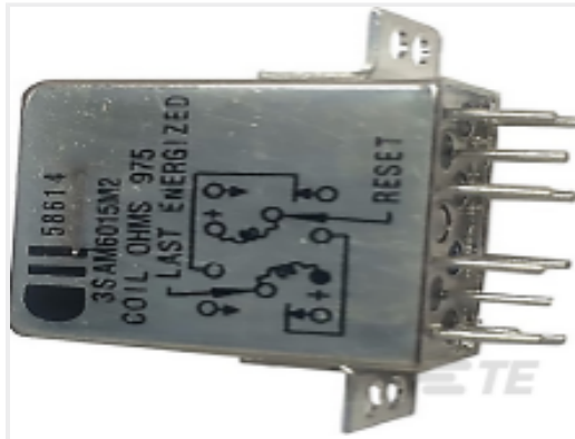
TE 产品编号 1617014-4 3SAT1307A2 = M5757/13-090
