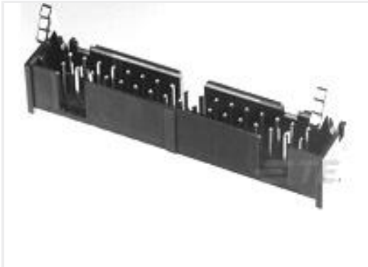
TE 产品编号3-1761608-7 IDC LOW PRO HDR 64P VERT SHT L
