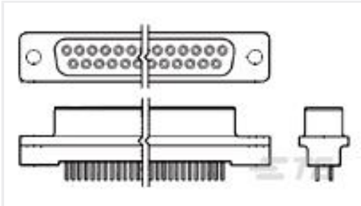
TE 产品编号207826-4 09 RCPT SP/AP STD
