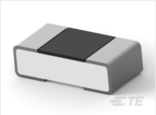
TE 产品编号6-2176363-7 RQ 0402 2K1 0.1% 10PPM 5K RL
