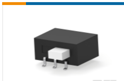
TE 产品编号1-1437581-1 ASE22RL=AUTOSLIDE DP 0.3W
