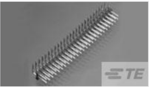
TE 产品编号 2-5176837-1 44 AMPMODU 2MM, H, AU, LF
