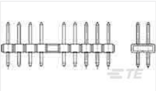
TE 产品编号 3-5176264-6 44 AMPMODU 2MM DR VERT MNT LF
