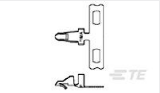
TE 产品编号350566-3 MINI AMP-IN 22-18 PTPBR
