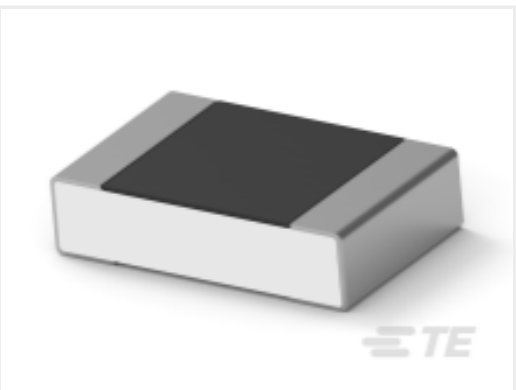
TE 产品编号2176373-5 RQ 0805 11R 0.1% 10PPM 1K RL
