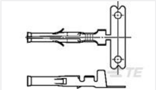
TE 产品编号350628-6 .062 COMM P&S SOK AUNI/PHBZ
