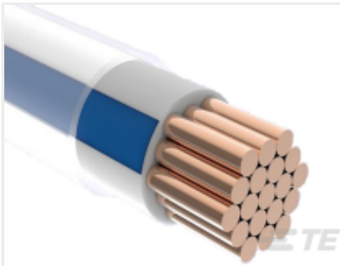
TE 产品编号CD78763001 ACW0219-1.00-41(NS)
