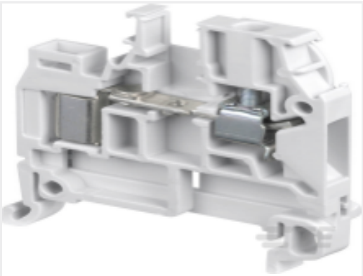
TE 产品编号 1SNA199555R2400 D2.5/5.ADO
