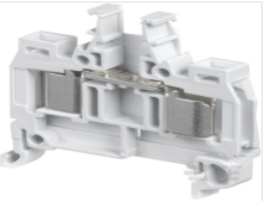
TE 产品编号 1SNA199083R1700 D1.5/6.ADO
