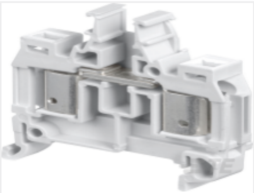
TE 产品编号 1SNA399318R1600 D4/8.N.ADO
