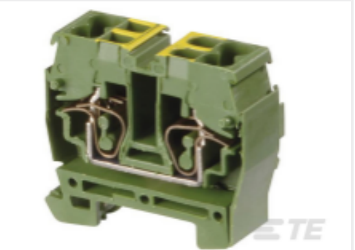
TE 产品编号1SNA290219R1200 DR2.5/10.P.4L
