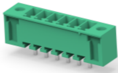
TE 产品编号 284516-6 6P TERMIBLOK HDR DIR C VITI
