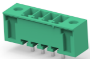
TE 产品编号 284516-4 4P TERMIBLOK HDR DIR C VITI
