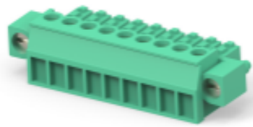
TE 产品编号 284511-9 9 POS TERMI-BLOK PLUG C. VITI
