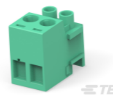
TE 产品编号 1986878-2 TERMI-BLOK PLUG 2 DIR 3.5MM MODULAR 2 P
