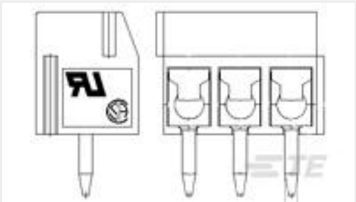
TE 产品编号1776275-3 3P TB ,90deg,VT,3.5mm,Blue,w /interlock
