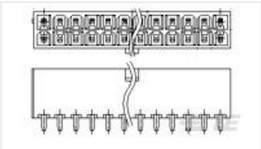
TE 产品编号4-1775099-5 ATX PWR CONN 14 POS
