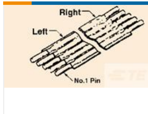
TE 产品编号5-1437141-1 FSN-22.5A-4= "FLXSTRP NMX .100
