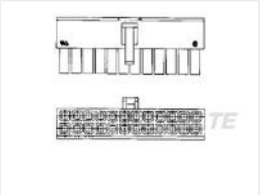
TE 产品编号1586019-8 8P RCPT VAL-U-LOK V0
