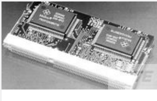
TE 产品编号6-390113-1 SKT,SODIMM,144P,SDRAM3.3V,STD, T&R
