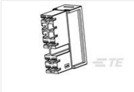
TE 产品编号 521978-2 HSG,RAST 5 PL,7P,B3,5,6,W/ VID
