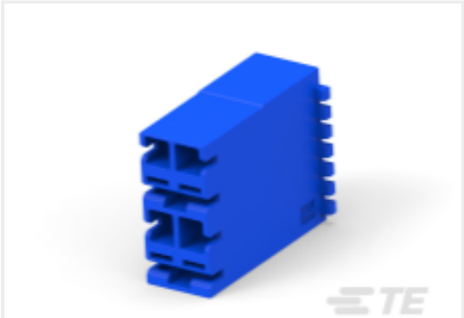
TE 产品编号 1969371-2 HSG, RAST 5 POSITIVE LOCK, 4P 2C
