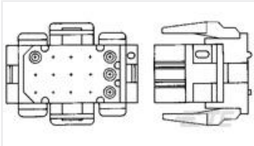
TE 产品编号205209-7 RECP ASSY SIZE 4
