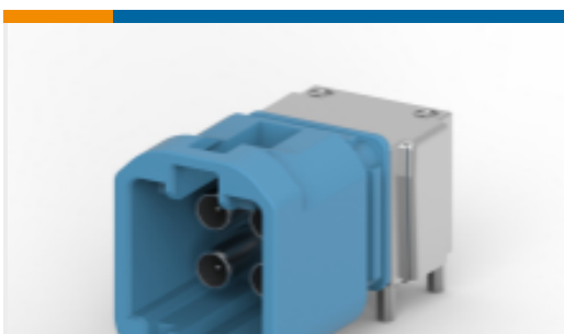
TE 产品编号2304168-3 4P MATE-AX, HDR ASSY,90 DEG,COD C
