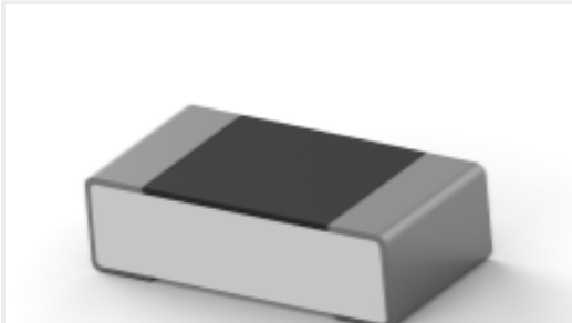
TE 产品编号4-2176369-7 RQ 0603 121R 0.1% 10PPM 5K RL
