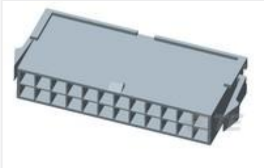
TE 产品编号1969605-2 2P PM PLUG VAL-U-LOK PM GW
