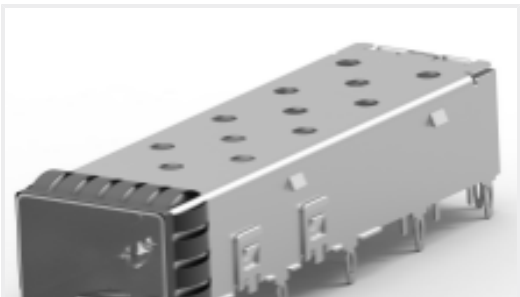
TE 产品编号 2007215-1 SFP+ 1x1 Cage Assy, PCI, Press
