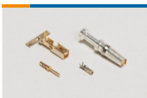
连接器端子(82)
