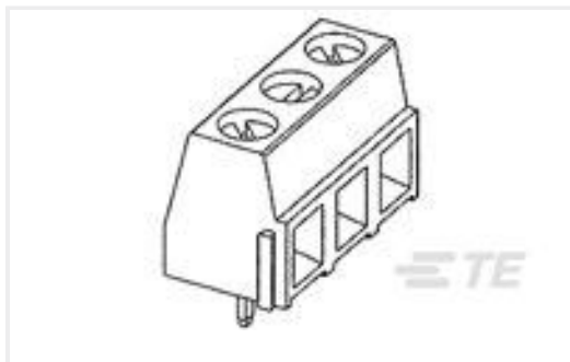
TE 产品编号 282837-5 TERMI-BLOK PCB MOUNT 5P
