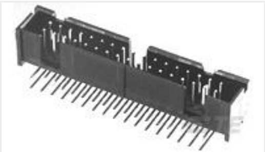
TE 产品编号103311-5 020 LOPRO HDR RA 30DP
