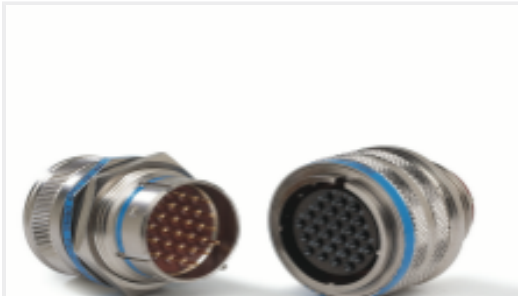
TE 产品编号ZPF000000000205570 DBAS 76G 61-21 SN 090-6117
